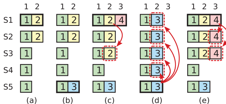
图 8: 图中的时序展示了为什么主员无法使用旧任期的日志条目来确定能否提交。在 (a) 中, S1 是主员, 部分复制了索引 2 处的日志条目。在 (b) 中, S1 崩溃了; S5 凭借 S3、S4 和它自己的投票当选为任期 3 的主员, 并在日志索引 2 处接受了一个不同的条目。在 (c) 中, S5 崩溃了; S1 重新启动, 被选为主员, 并继续复制。此时, 来自任期 2 的日志条目已在多数服务器上复制, 但尚未提交。在 (d) 中, 如果 S1 又崩溃了, S5 可以当选主员 (有 S2、S3 和 S4 的投票), 并用它自己的任期 3 的条目覆盖 S1 的条目。然而, 如果 S1 在崩溃之前将其当前任期的条目复制到了多数服务器上, 如 (e) 中所示, 那么该条目就提交了 (S5 无法赢得选举)。此时, 日志的所有先前条目也会提交。
