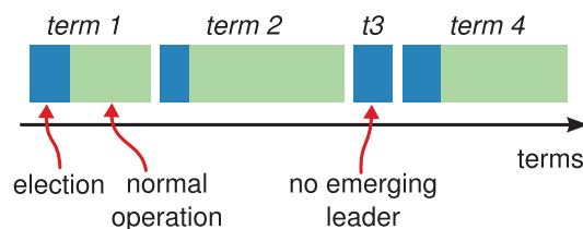
图 5: 时间划分为任期, 每个任期都始于选举。选举成功后, 由一个主员管理集群, 直到任期结束。有些选举失败了, 这种情况下, 任期结束但没有主员。不同的服务器可能在不同的时刻观察到任期转换。
