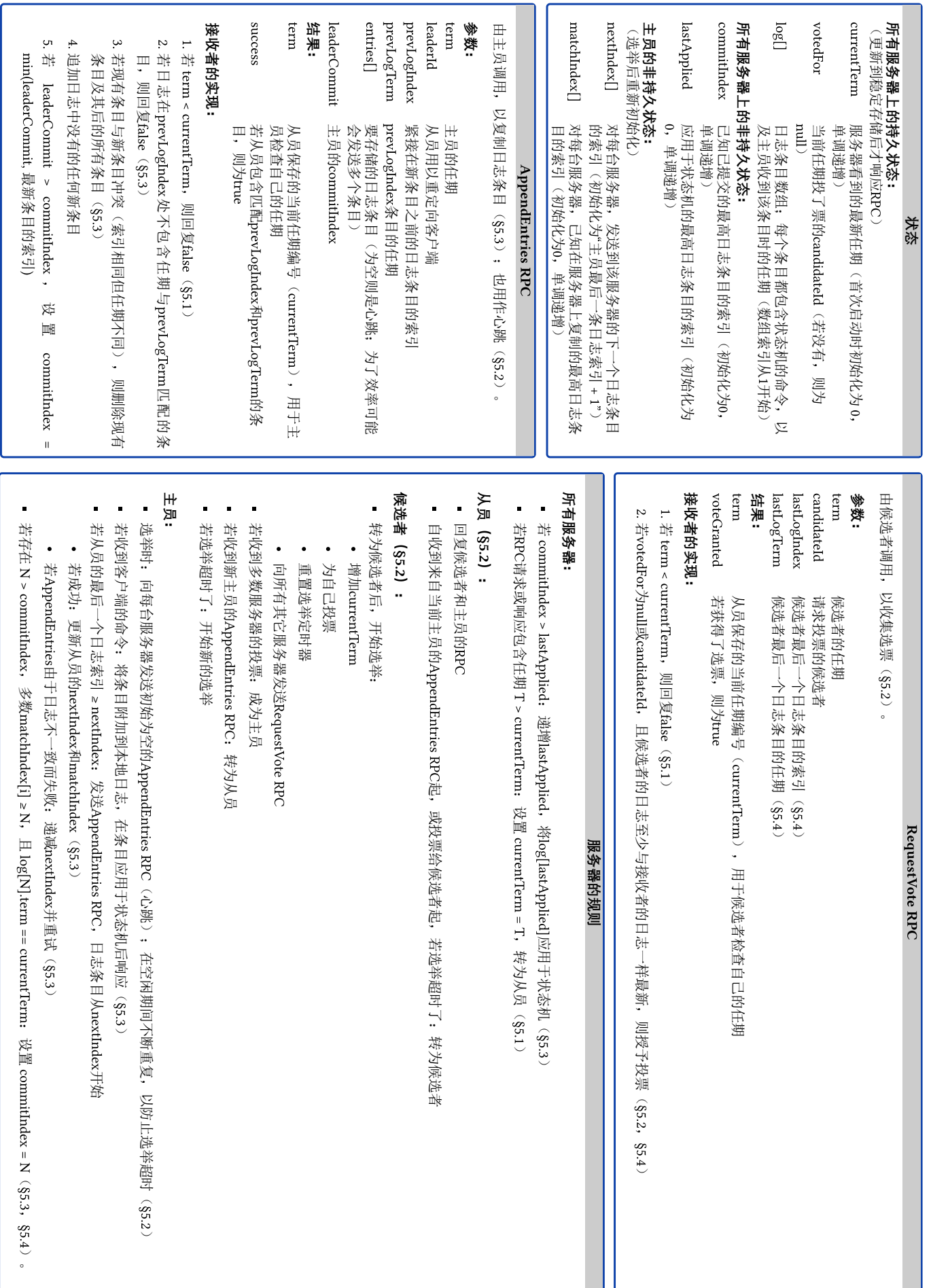
图 2: Raft 共识算法的简要总结 (不包括成员变更和日志压缩)。左上框中的服务器行为被描述为一组独立且重复触发的规则。§5.2 等小节编号表示本文中讨论特定功能的位置。形式化规范 [31] 更准确地描述了该算法。
