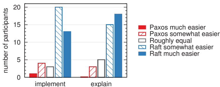
图 15: 使用 5 分制，参与者被问及（左）他们认为哪种算法更容易在功能正常、正确且高效的系统中实现，以及（右）哪种算法更容易向计算机科学专业的研究生解释。
