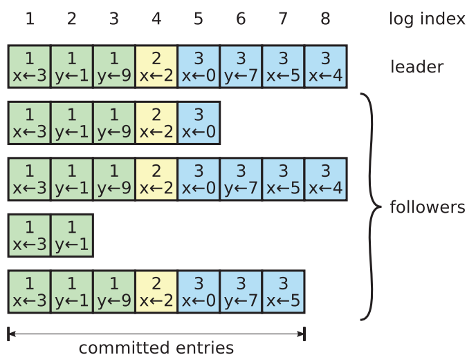
图 6: 日志是由条目组成的, 这些条目按顺序编号。每个条目都包含创建它的任期(框中的数字)和状态机的命令。若条目可以安全地应用于状态机, 则认为该条目已提交。
